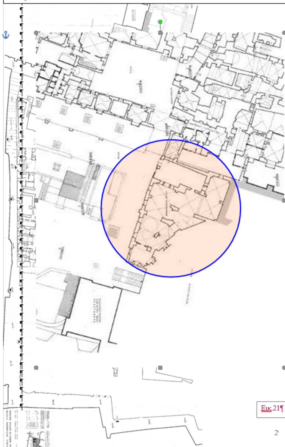
Τοπογραφική αποτύπωση του μοναστηρίου των αγίων Κωνσταντίνου και Ελένης· Ground floor
